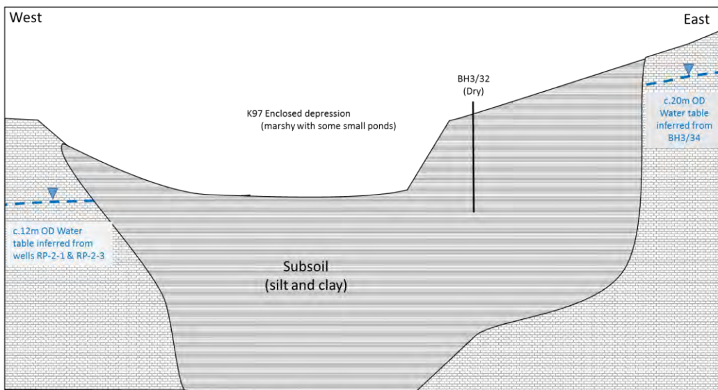
Pláta 10.10 Scéimléaráid de thrasghearradh soir siar trí Logán lata K97 a léiríonn Idirghníomhú an Screamhuisce leis an nGné le linn Ardleibhéal Screamhuisce
