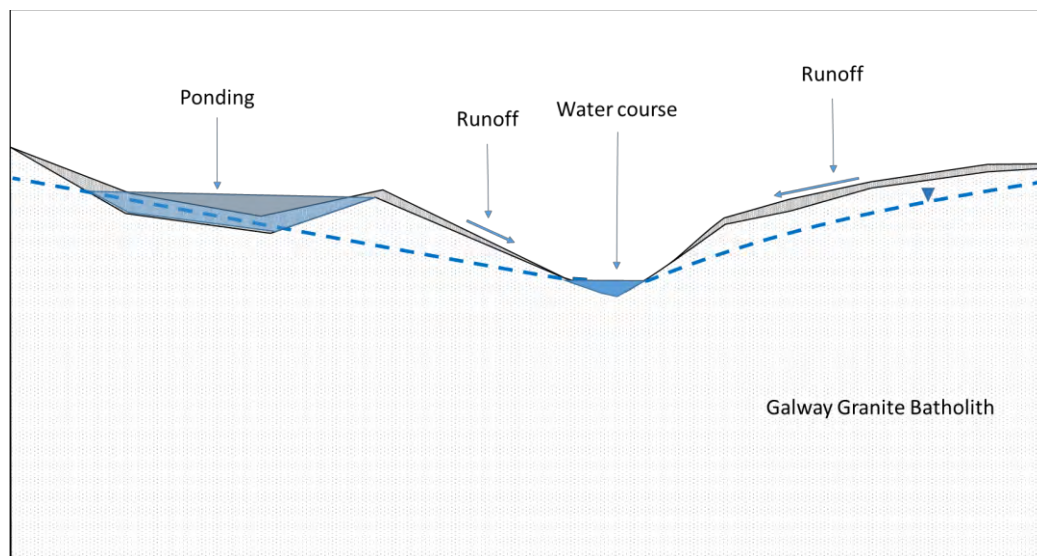
Pláta 10.2 Coincheapú Hidrigeolaíochta ar Rith Chun Srutha agus Carnadh Uisce Dromchla ar Bhatailit Eibhir na Gaillimhe
