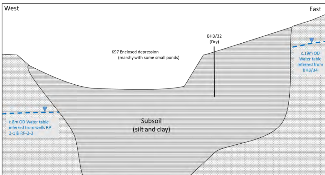
Pláta 10.11 Scéimléaráid de thrasghearradh soir siar trí Logán lata K97 a léiríonn Idirghníomhú an Screamhuisce leis an nGné le linn Leibhéal Ísle Screamhuisce
