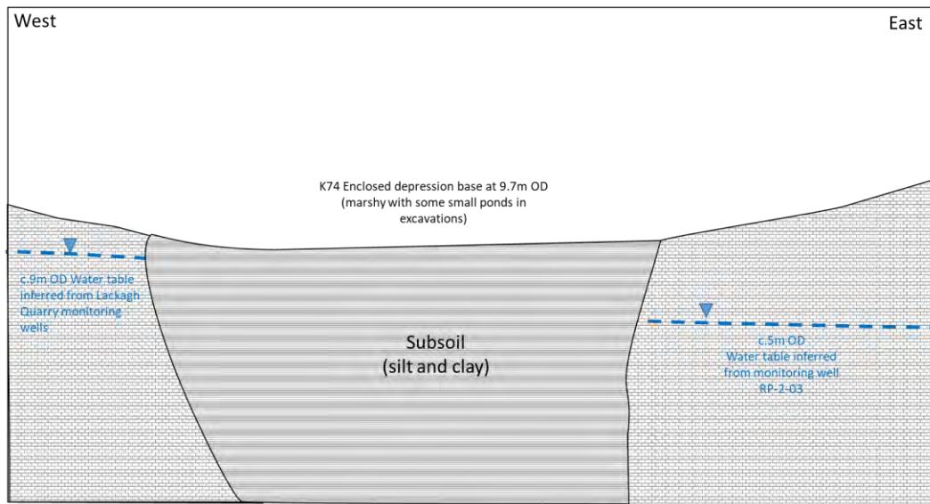
Pláta 10.13 Scéimléaráid de thrasghearradh soir siar trí Ghné a léiríonn Idirghníomhú an Screamhuisce leis an nGné le linn Leibhéal Ísle Screamhuisce
