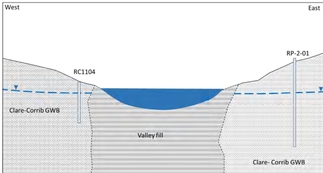
Pláta 10.8 Scéimléaráid de thrasghearradh soir siar trí Loch an Dúlaigh a léiríonn Idirghníomhú an Screamhuisce leis an Loch le linn Leibhéal Ísle Screamhuisce
