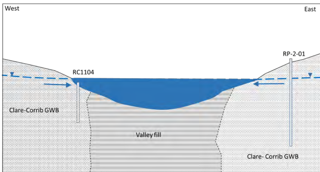
Pláta 10.7 Scéimléaráid de thrasghearradh soir siar trí Loch an Dúlaigh a léiríonn Idirghníomhú an Screamhuisce leis an Loch le linn Ardleibhéal Screamhuisce
