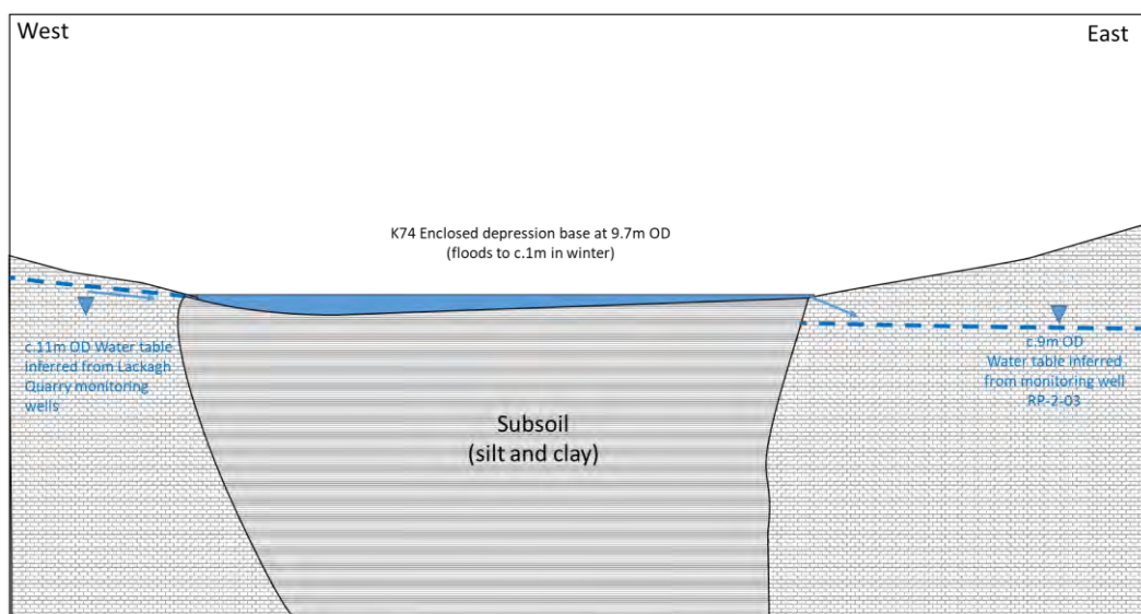
Pláta 10.12 Scéimléaráid de thrasghearradh soir siar trí Ghné a léiríonn Idirghníomhú an Screamhuisce leis an nGné le linn Ardleibhéal Screamhuisce
