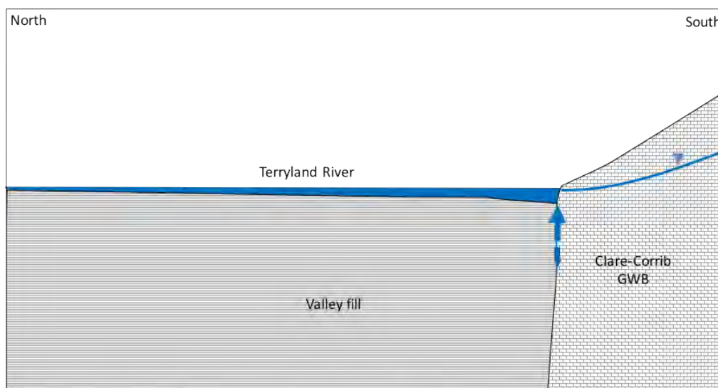
Pláta 10.14 Scéimléaráid de thrasghearradh thuaidh theas trí Abhainn Thír Oileáin ag léiriú Oibriú na Estavelles ag Poll an Mhuirín Thiar agus Thoir le linn Ardleibhéal Screamhuisce
