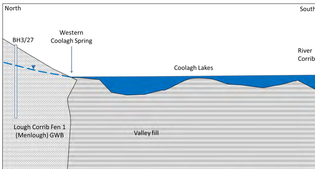
Pláta 10.3 Trasghearradh scéimreach thuaidh theas trí Lochanna Chúil Each (Screamhuisce Ard)
