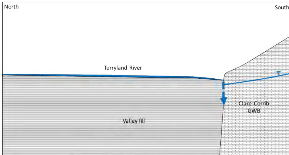
Pláta 10.15 Scéimléaráid de thrasghearradh thuaidh theas trí Abhainn Thír Oileáin ag léiriú Oibriú na Estavelles ag Poll an Mhuirín Thiar agus Thoir le linn Leibhéal Screamhuisce
